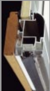
Doble sistema cortavientos Double system wind breaker Double system coupe-vent
